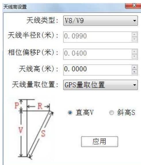
图 18-7 天线高设置
