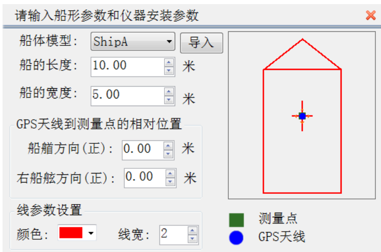
图 9-1 船形设计
