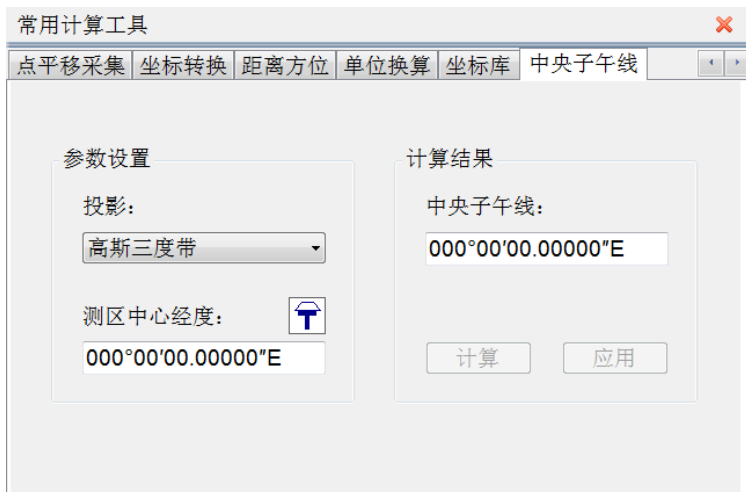
图 19-23 中央子午线
