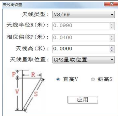
图 8-15 天线高计算
