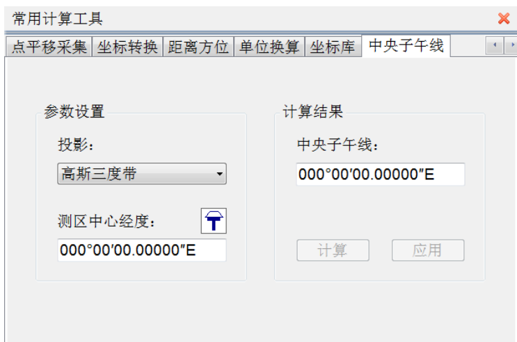
图 19-23 中央子午线
