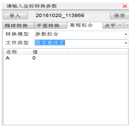
图 7-11 固定差改正
