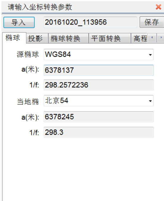
图 7-3 椭球参数
